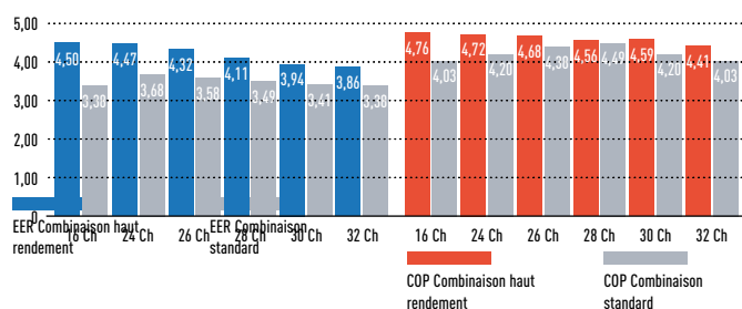
EER/COP (W/W) COP leader du marché (à pleine charge), combinaison haut rendement
