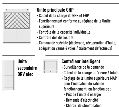
Schéma du système hybride GHP/DRV élec
