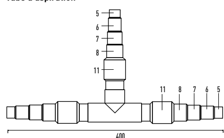
Tube d'aspiration
