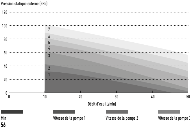
Performance de la pompe hydraulique pour les pompes à chaleur de type F : pompe de classe A, type F (5kW et 16kW).
