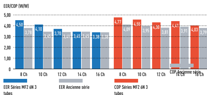
COP leader du marché (à pleine charge), efficacité standard.
